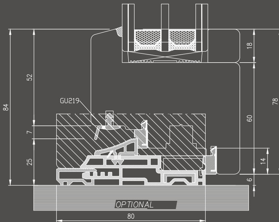
Nodo inferiore portafinestra con soglia
