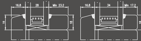
Junquillo Tipo 3 (Cuadrado)
