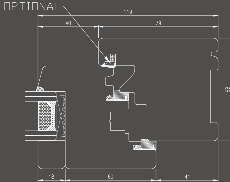
Galce superior/lateral ventana y balconera
