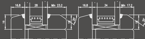
Junquillo Tipo 2 (Achaflanado)
