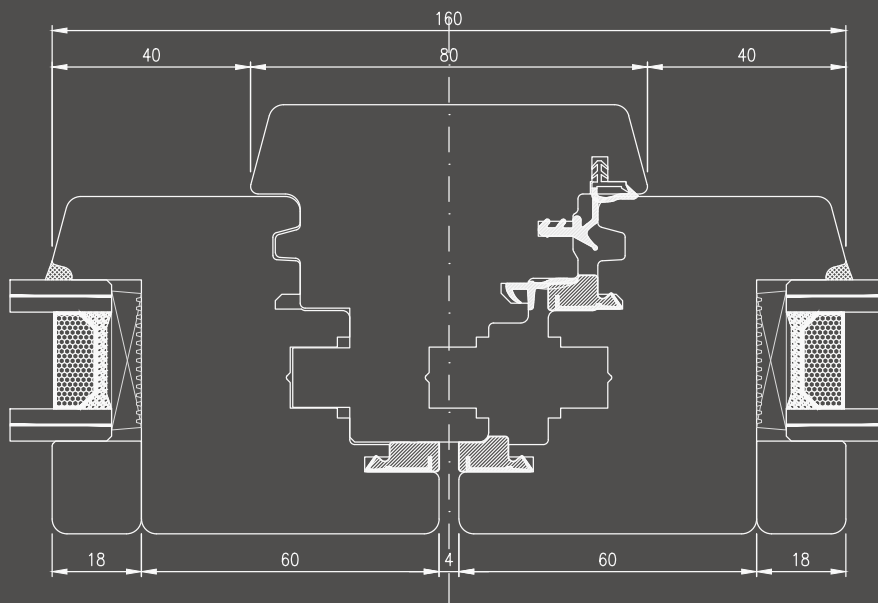
A9 Galce central de ventanas y balconeras
