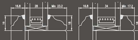
Junquillo Tipo 4 (Barroco)
