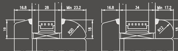
Junquillo Tipo 1 (Redondeado)
