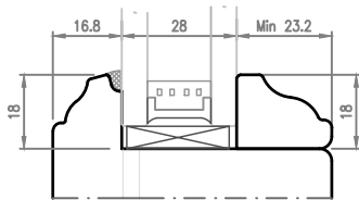
Fermavetro Tipo 4 (Barocco)
