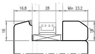
Fermavetro Tipo 2 (Smussato)
