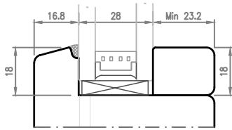
Fermavetro Tipo 3 (Squadrato)
