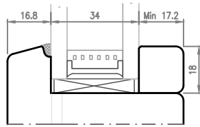
Fermavetro Tipo 3 (Squadrato)
