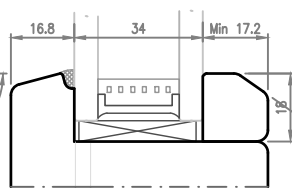
Fermavetro Tipo 2 (Smussato)
