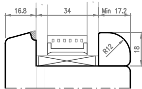
Fermavetro Tipo 1 (Arrotondato)
