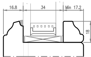
Fermavetro Tipo 4 (Barocco)
