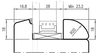
Fermavetro Tipo 1 (Arrotondato)
