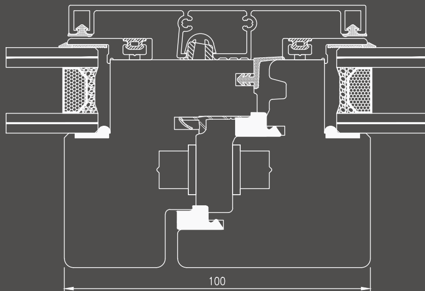
Galce central de ventana/balconera
