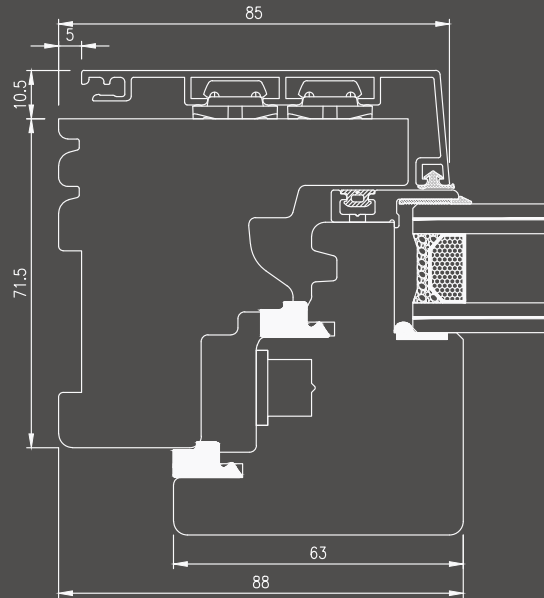
Galce superior/lateral ventana y balconera
