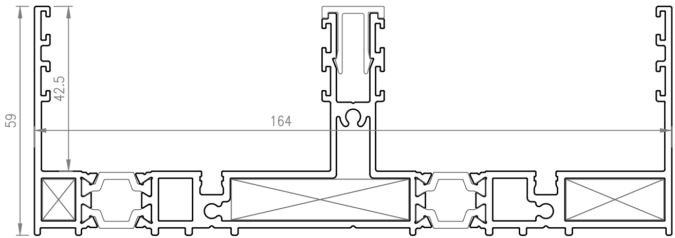
Telaio inferiore e laterale
