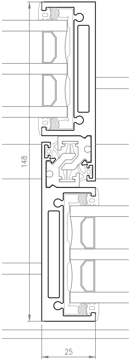
Nodo centrale standard
