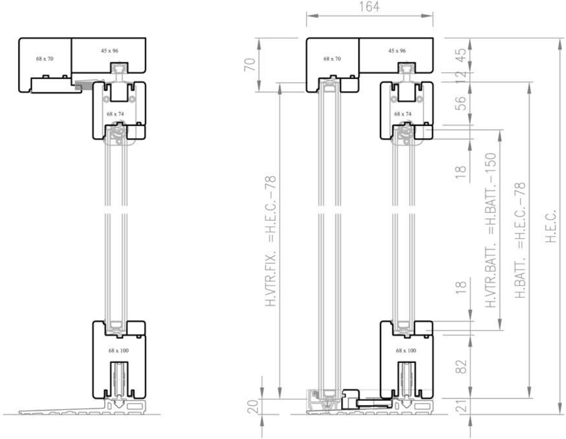
SEZ. VERTICALE
