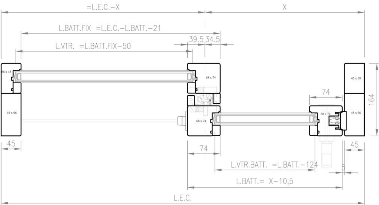
SEZ. ORIZZONTALE
